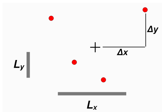
図 16-2：格子点 (+) でのデータ値 (赤い記号) の加重平均。詳細は本文を参照してください。
