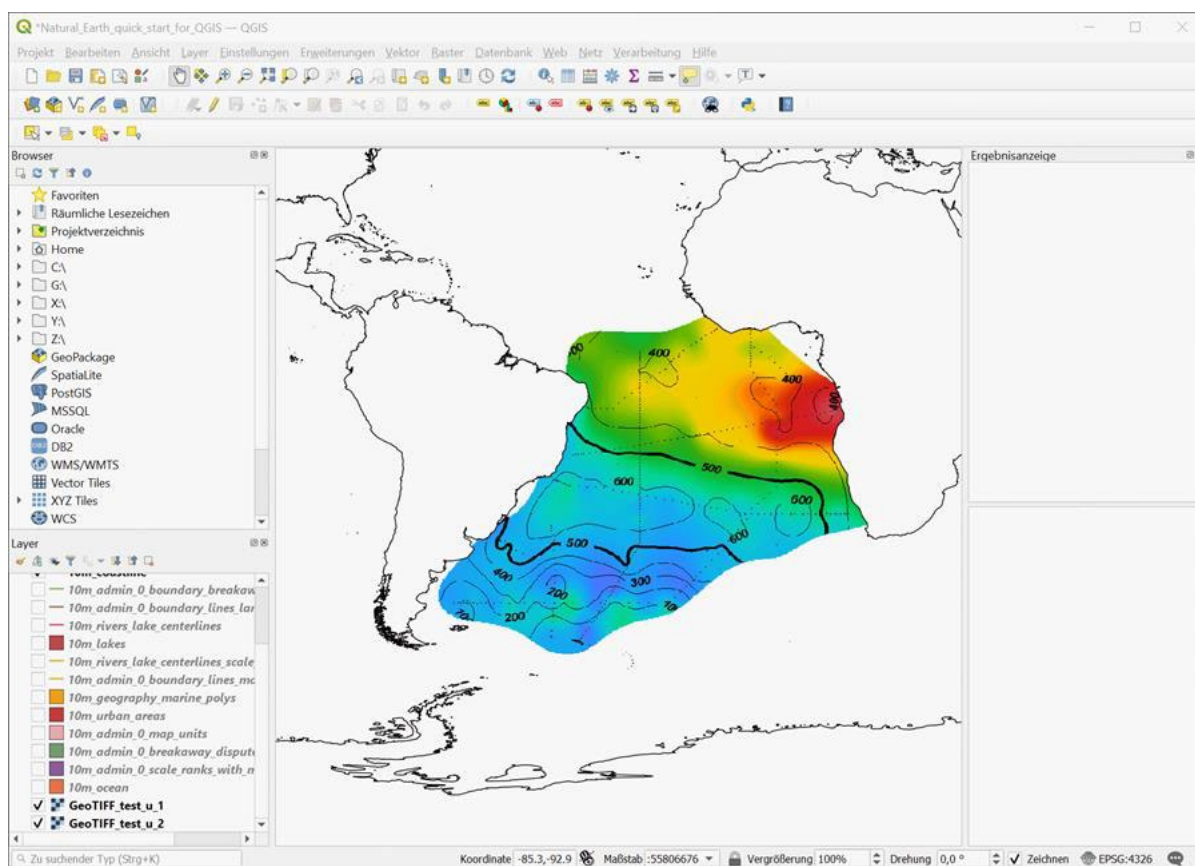
図 1-8: \sigma_0=27.0 の等密度面の等深線および色付けされた同じ等密度面上でのリン酸塩濃度の GIS での表示例
